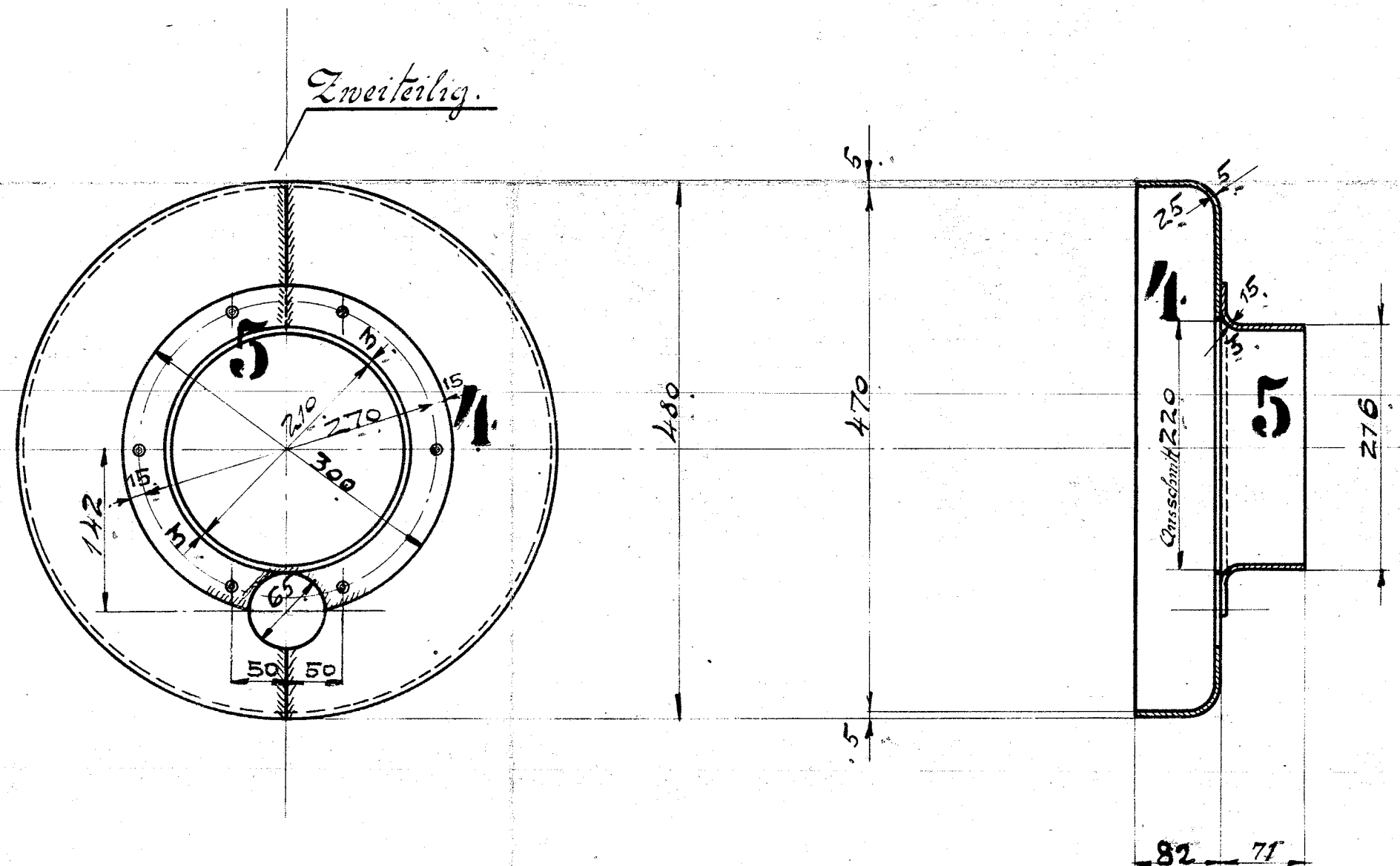
Behleidungshappe für vord. Cylinderdeckel.
