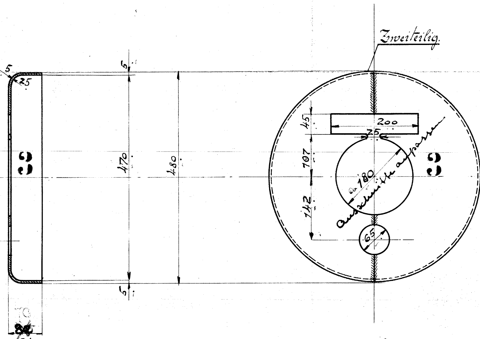
Behleidungshappe für hint. Cylinderdeckel.
