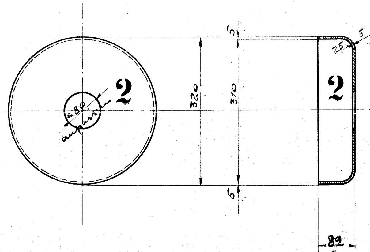
Behleidungshappe für vord. Schieberkasten deckel.
